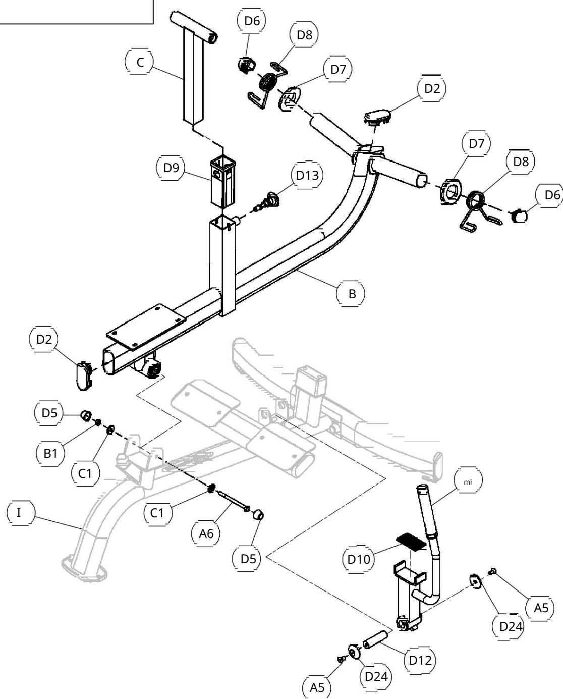
Krok 2: Zakończenie montażu
