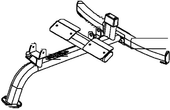
Krok 1: Zakończenie montażu
